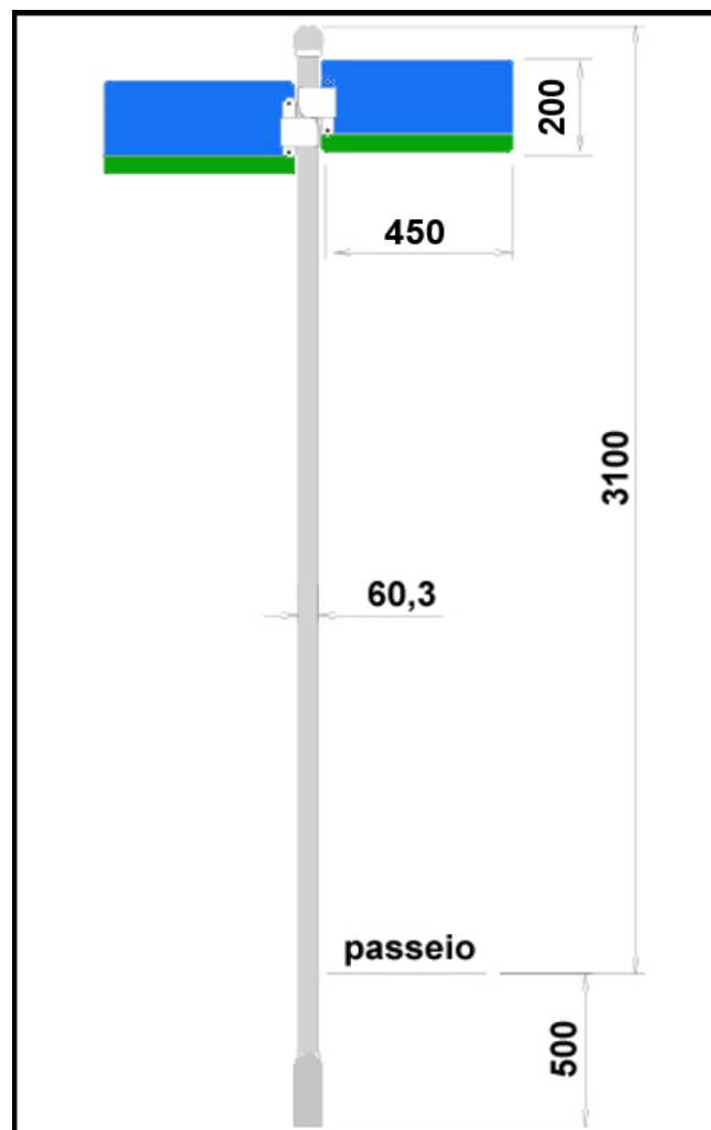
Ilustração 2: Detalhe do poste (medidas em mm)
