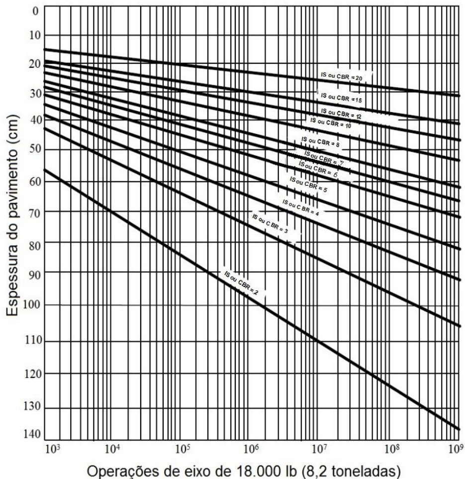
Ilustração 1: Ábaco para dimensionamento de espessuras de pavimentos
