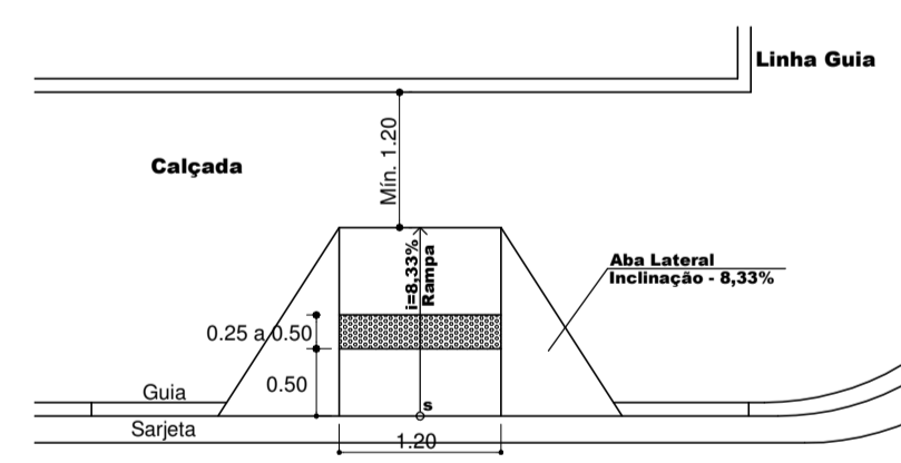
Detalhe Rabaixamento em calçada larga
