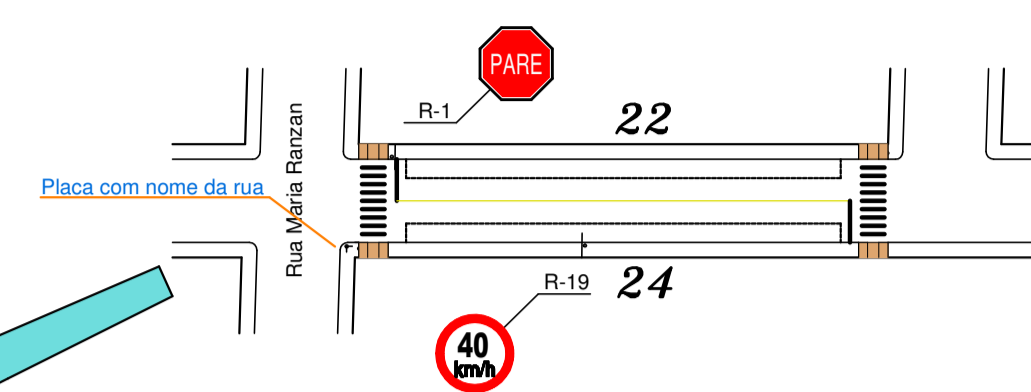
Rua Alberto Tressoldi Escala: 1:1.000
