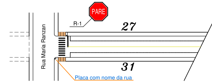
Rua Ortenila Bortolanza Escala: 1:1.000
