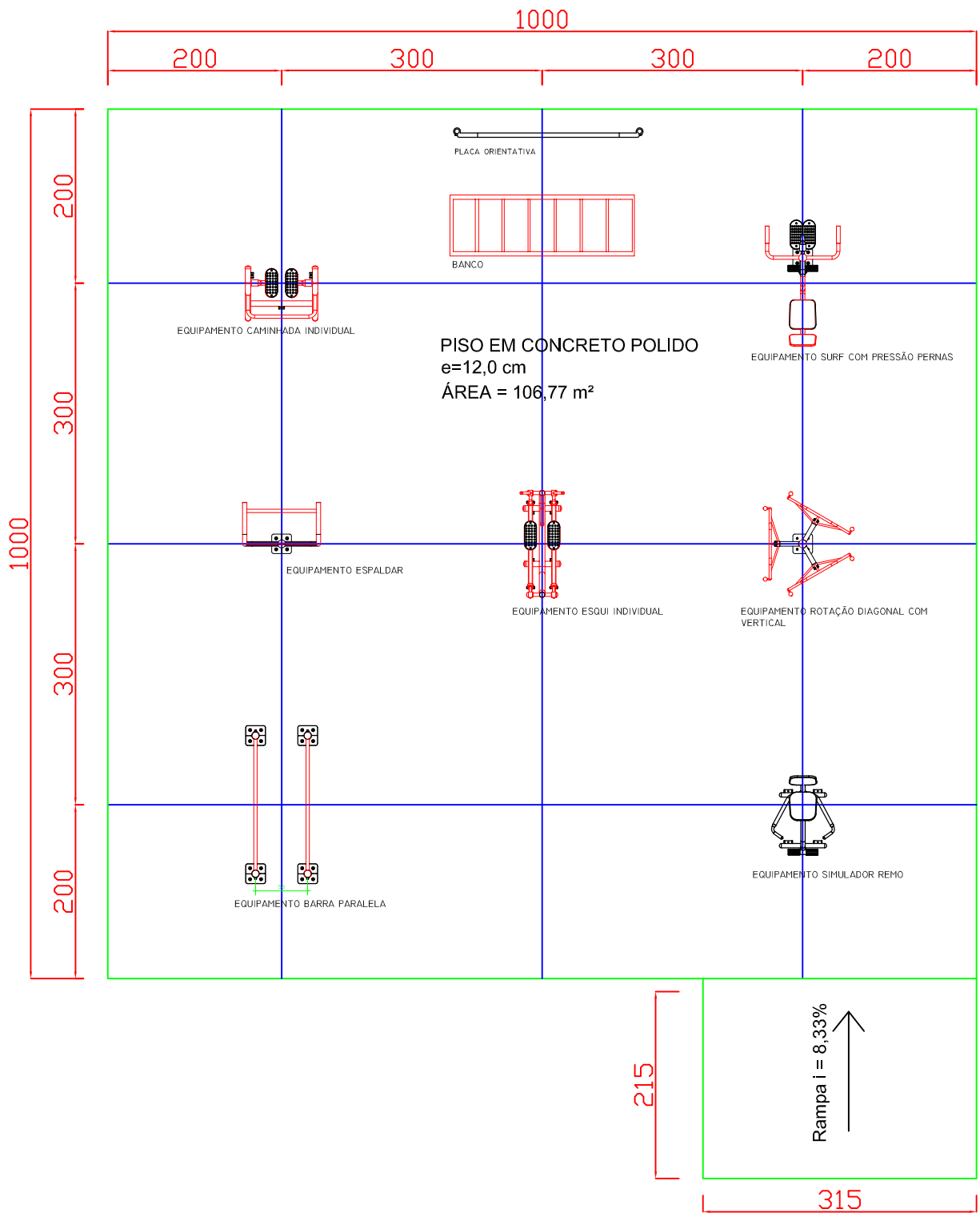
PLANTA BAIXA ACADEMIA - BAIRRO ROSA LINDA ÁREA: 106,77 m 2 ESCALA: S/E
