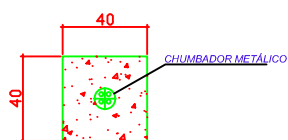
DETALHE CHUMBADORES DOS BRINQUEDOS PLANTA BAIXA S/E.
