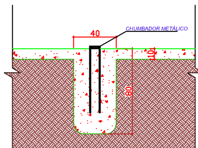
DETALHE CHUMBADORES DOS BRINQUEDOS CORTE ESQUEMÁTICO S/E.
