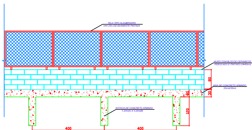
DETALHE FECHAMENTO LATERAL DO PARQUE CORTE ESQUEMÁTICO S/E.
