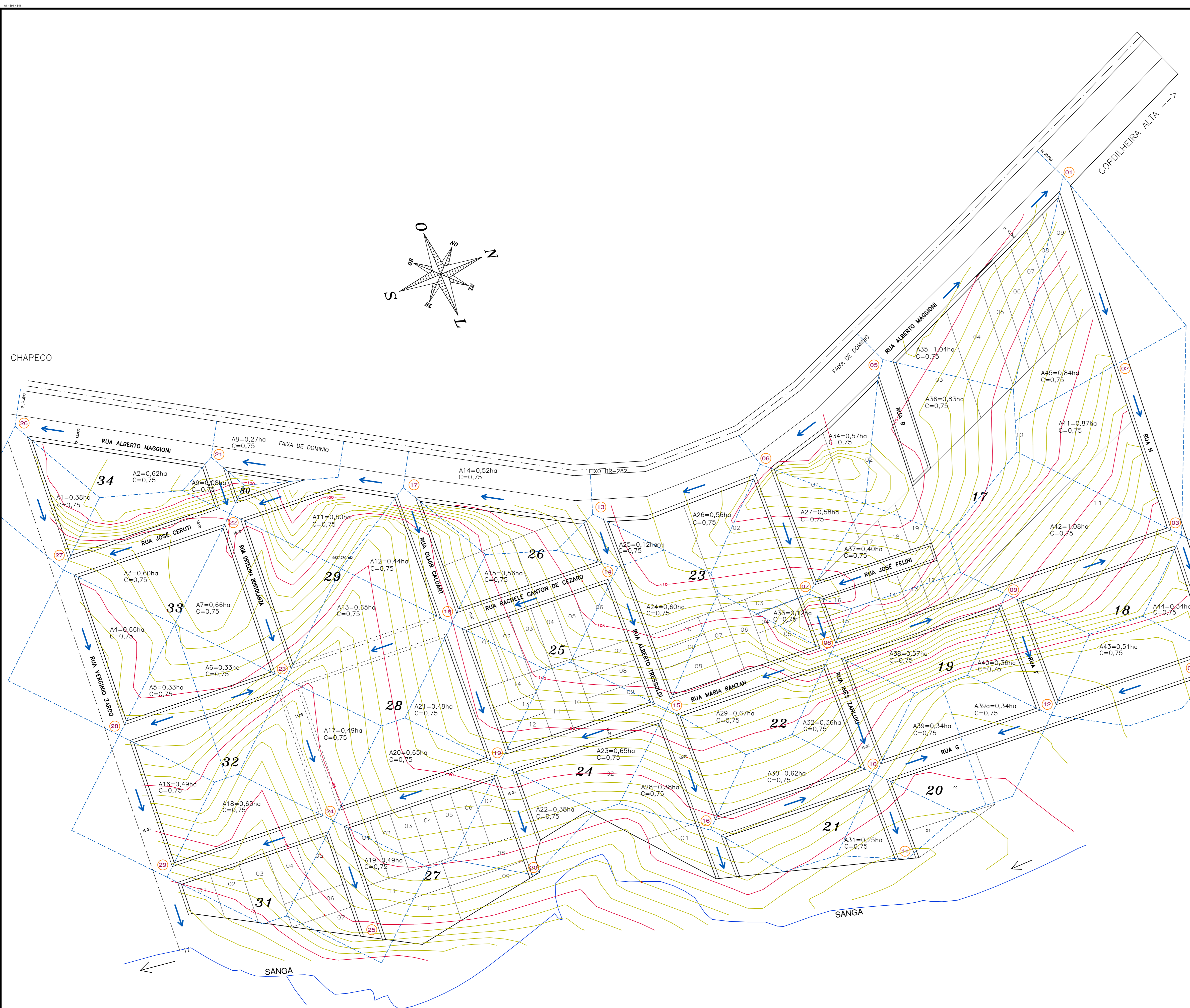
Planialtimétrico e áreas de contribuição Escala: 1:1.250
