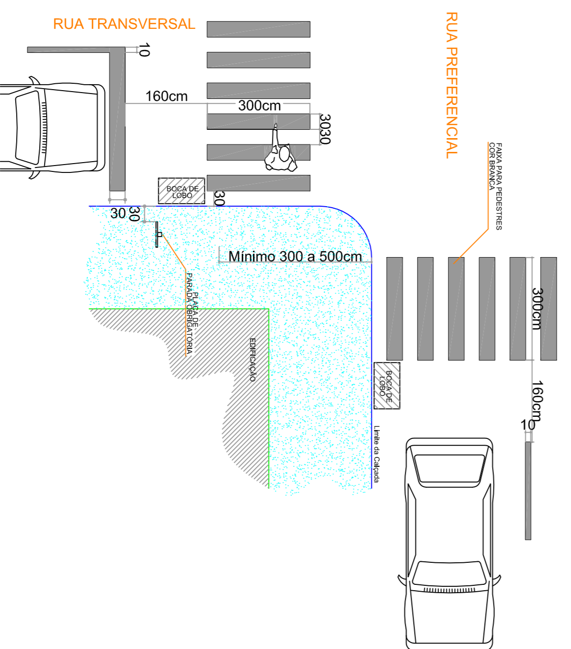
DETALHE 1 POSICIONAMENTO DA PLACA DE PARADA OBRIGATORIA EM RELAÇÃO À ESQUINA E FAIXA PARA PEDESTRES
